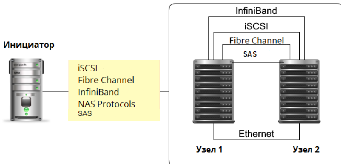
Рис. 2 ПО RAIDIX: Двухконтроллерный режим работы
